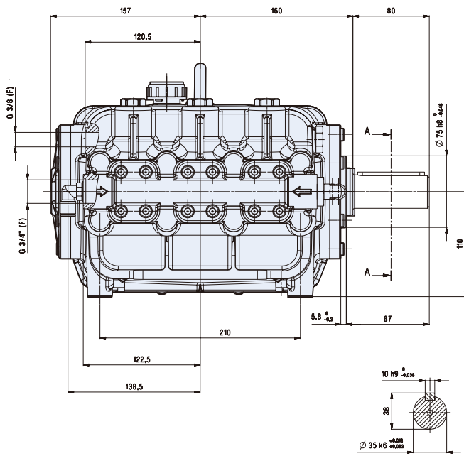
SEZ. A-A
