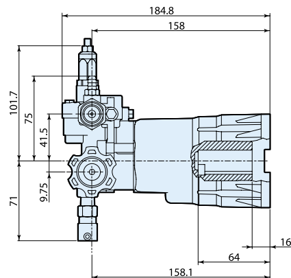
铝泵头
